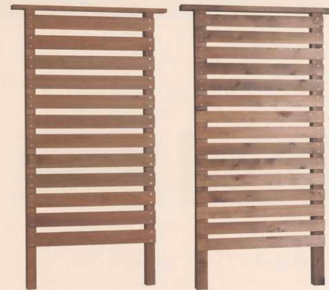
素材:天然堅木(左)/米杉(右) サイズ:高さ1,800mm×柱間1,000mm
